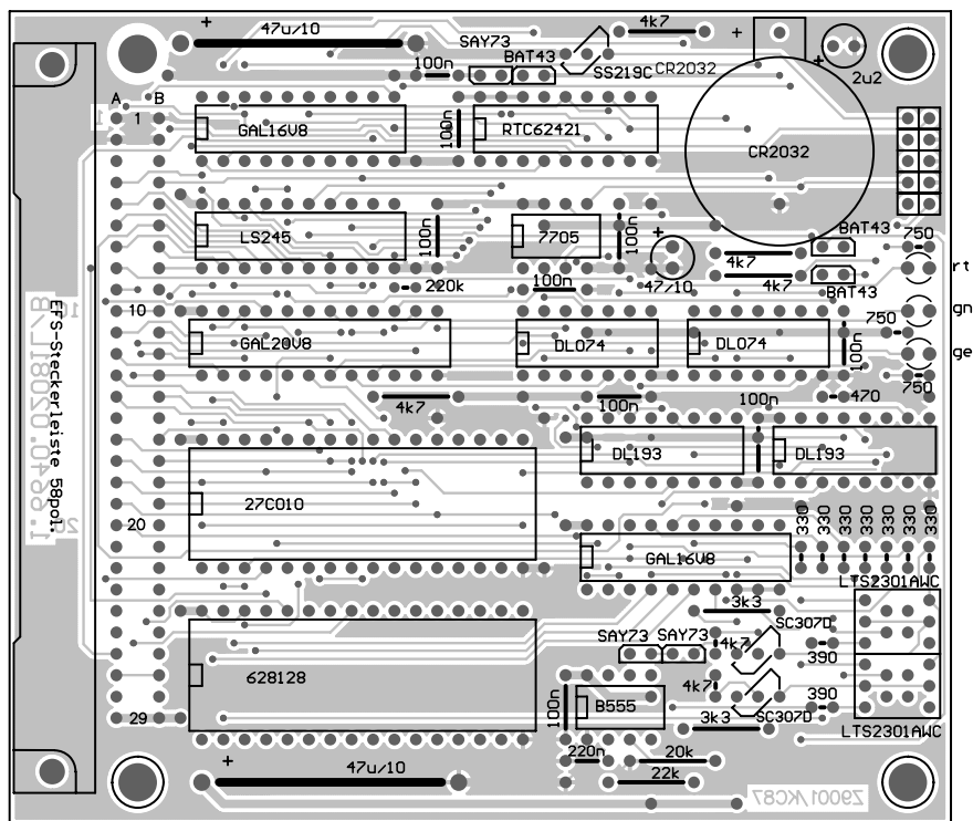
Top Overlay
