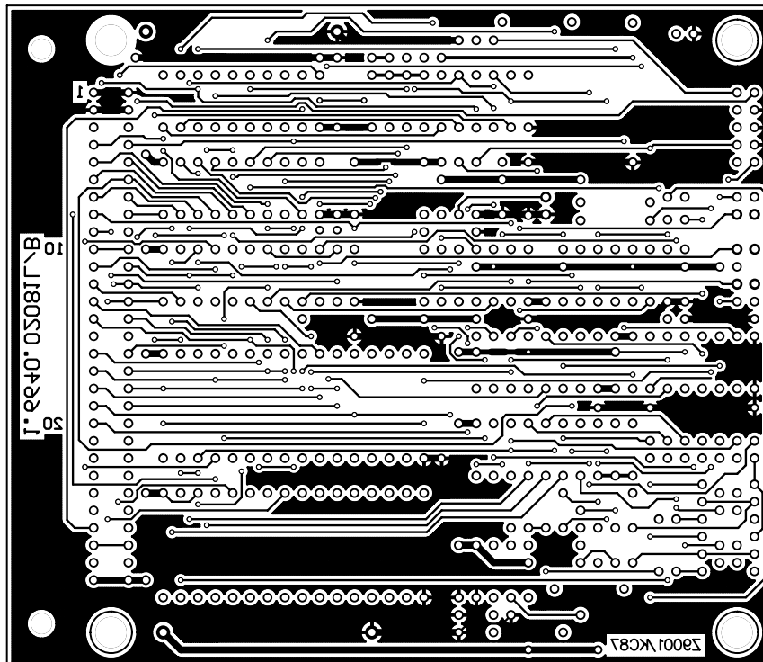
Bottom Layer
