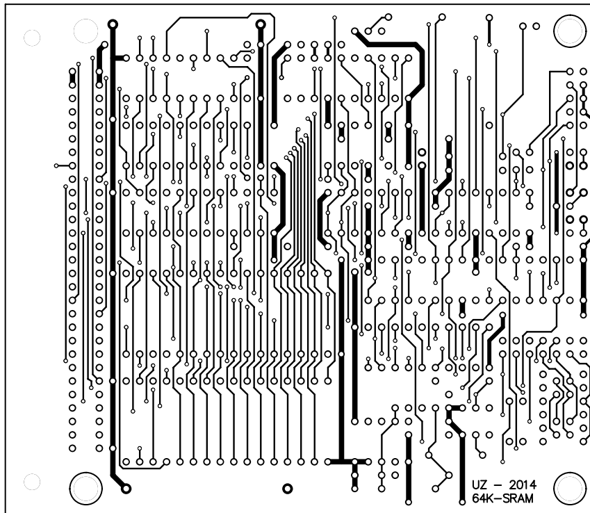
Top Layer
