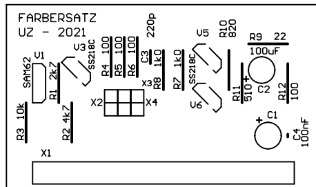
Top Overlay
