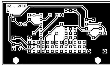
Bottom Layer
